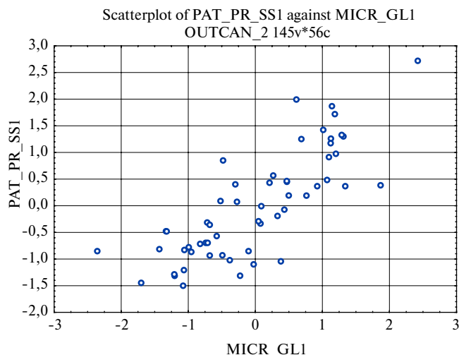
Рис. 1. Графическое представление результатов канонической корреляции. Примечание: вертикальная ось (PAT_PR_SSI) — отражает совокупность 14 признаков, характеризующих изменения в КА (количество диагональных ветвей ПНА, количество септальных ветвей ПНА, количество стенозов в ОА, количество стенозов в ПКА, количество стенозов более 70% в ОА, количество стенозов более 70% в ПКА, максимальный процент стеноза в ОА, максимальный процент стеноза в ПКА, количество патологических процессов, выявленных в КА, общее количество стенозов во всех КА, общее кол-во КА со стенозами, общее количество КА с кальцинозом, общее количество КА с острым тромбозом, общее количество КА с протяженными стенозами); горизонтальная ось (MICR_GLI) отражает совокупность 7 признаков, характеризующих параметры микроциркуляции (средние значения АВК, среднее количество капилляров на 1 \text{ мм}^2 поверхности конъюнктивы, распространенность ВСАЭ в зоне угла глаза, распространенность ВСАЭ в центральной зоне бульбарной конъюнктивы, распространенность ВСАЭ в переходной зоне бульбарной конъюнктивы, распространенность ВСАЭ в зоне перилимба, количество зон конъюнктивы с выявленной ВСАЭ).
